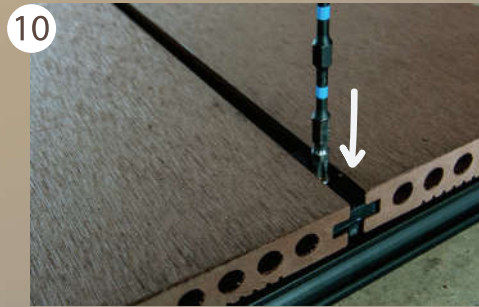
ยังยึดลงบนตงด้วยสกรูสแตนเลสตามแนวตง
