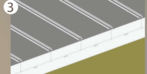
ติดตั้งตะแกรงเหล็กฉวาลายไม้/ตะแกรง WPC ยึดลงบนพื้นคอนกรีต เว้นระยะสเปก 30-40 เซนติเมตร
