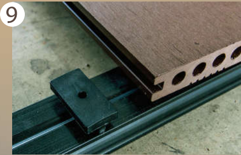
กรณีต้องการเว้นร่องระหว่างแผ่นให้มากขึ้น (4-5 มม.) ให้ใช้คลิปเว้นร่องห่าง วางระหว่างแผ่นไม้พื้น 2 แผ่น
