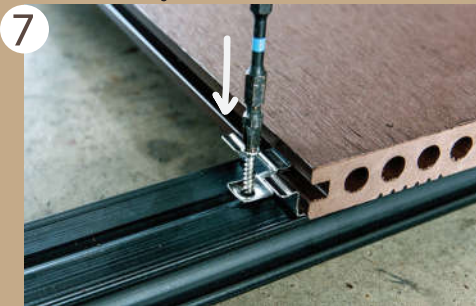
ยึดคลิปเข้ากับตงด้วยสกรูสแตนเลสลงบนตงตามแนว
