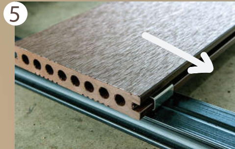
เลื่อนแผ่นไม้พื้นเข้าประกบกับคลิปตัวเริ่ม
