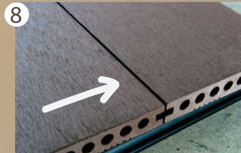
สอดแผ่นไม้พื้นแผ่นต่อไปเข้ากับร่องคลิป (จะปรากฏร่องระหว่างแผ่นไม้พื้นประมาณ 1 มม.)
